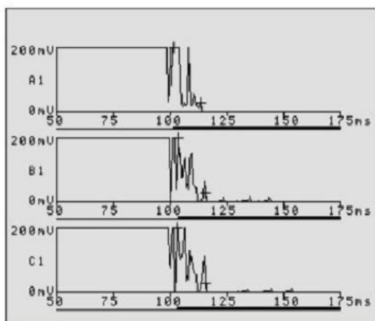
合闸动态电阻波形
