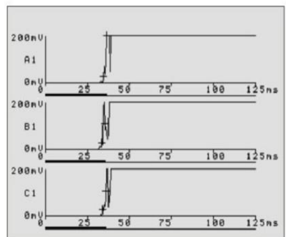
分闸动态电阻波形
