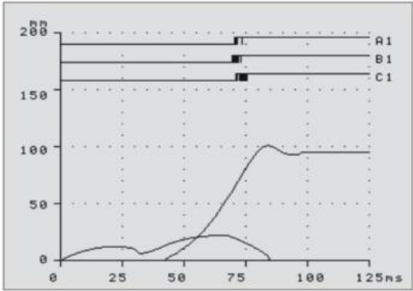
合闸测试图形
