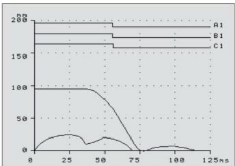
合--分闸测试图形
